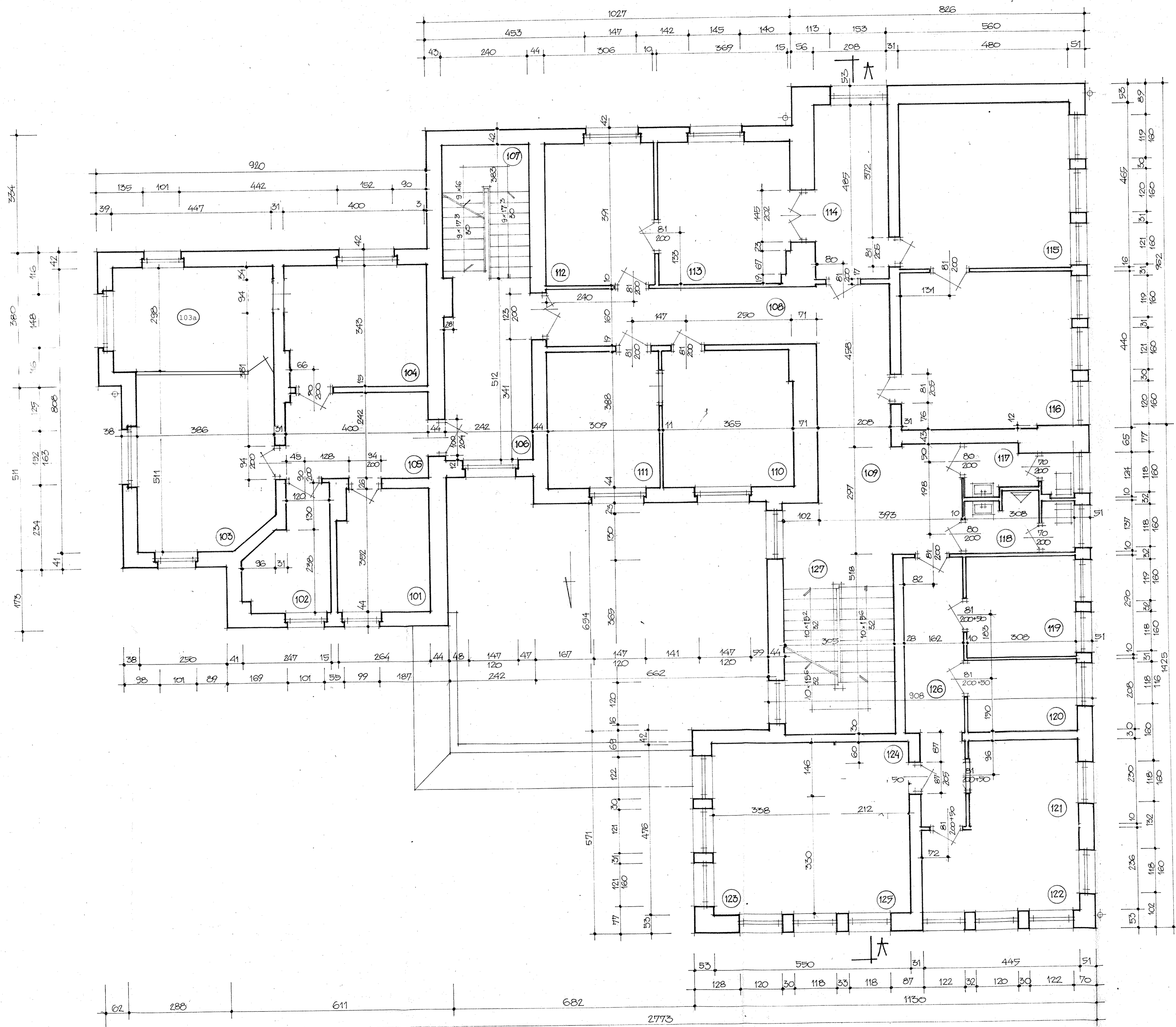
RZUT I PIĘTRA - SKALA 1:50
