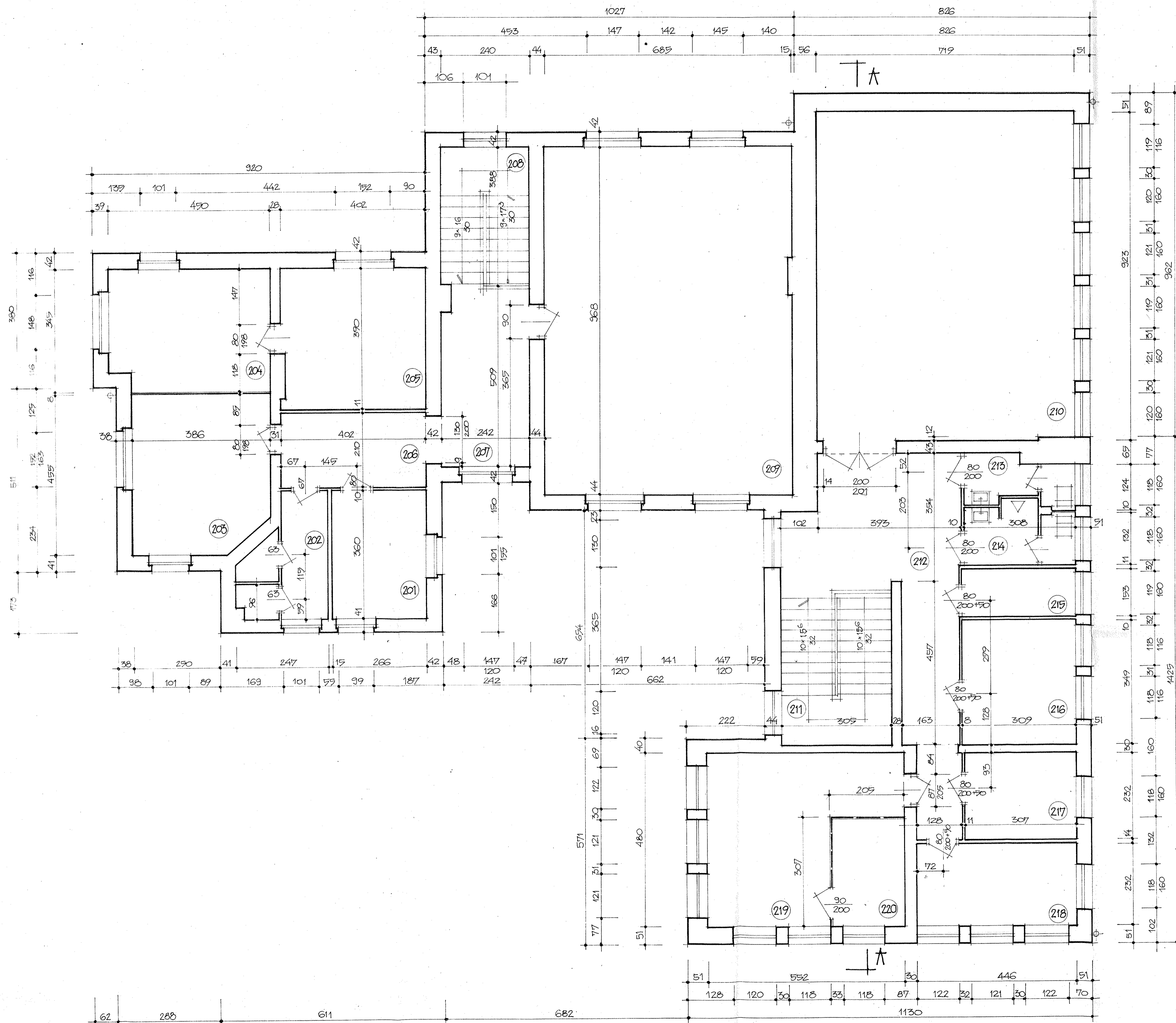
RZUT II PIĘTRA - SKALA 1:50
